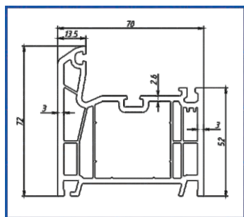
Профиль рамы Frame
