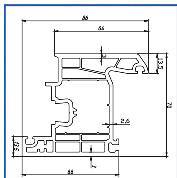
Профиль створки Sash
