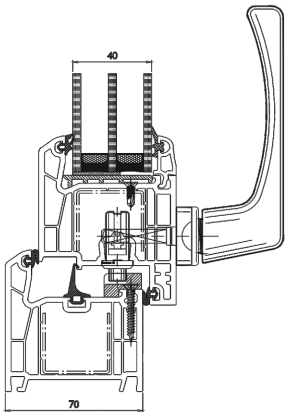
Монтаж профиля рамы и створки серии 70 мм
