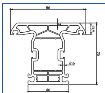
Профиль импоста Transom
