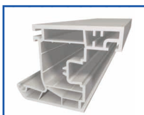
Профиль створки Sash
