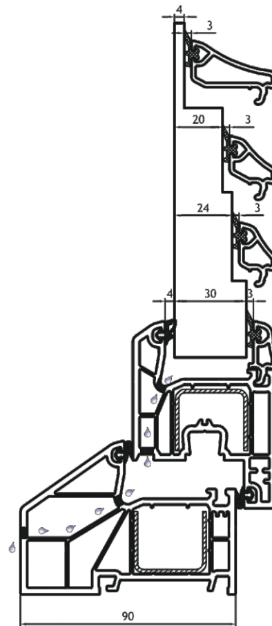
Стеклопакет 30 мм. Штапик 3-00-03-19-****
