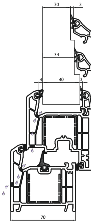
Стеклопакет 30 мм. Штапик 3-00-03-19-****
