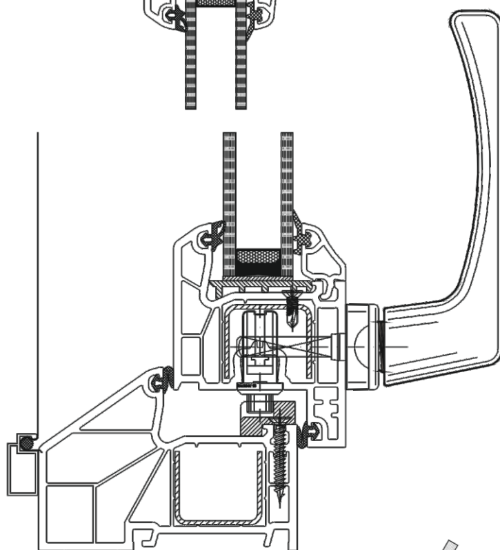
Монтаж профиля рамы thermo и створки
