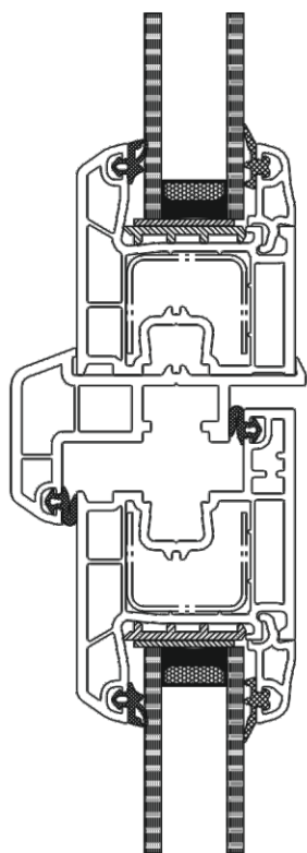
Монтаж адаптера активной створки серии 53 мм
