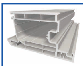
Дверной профиль наружного открывания Outward Opening Door
