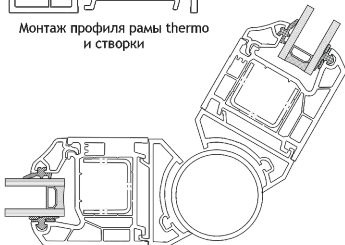
Монтаж углового трубчатого соединительного профиля
